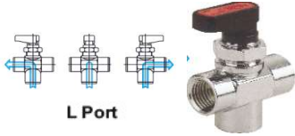
6700 - Küresel 3 Yol
