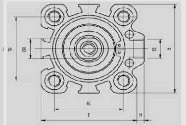
BB/BF 32 - 100
