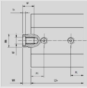
BB/BF 32 - 100
